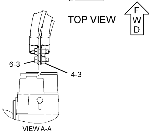
VIEW A-A
